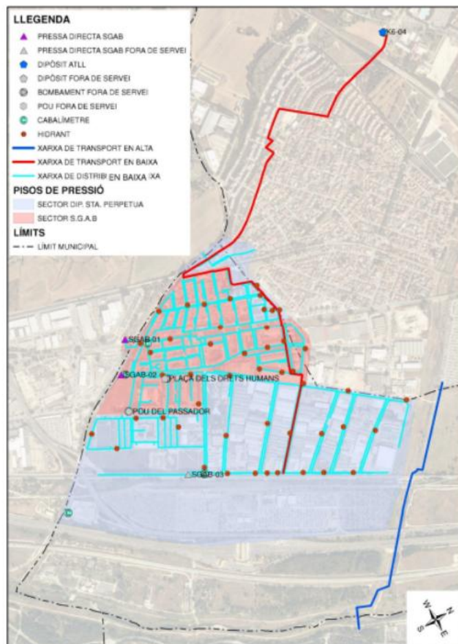
Esquema general del sistema d'abastament de la Llagosta.
